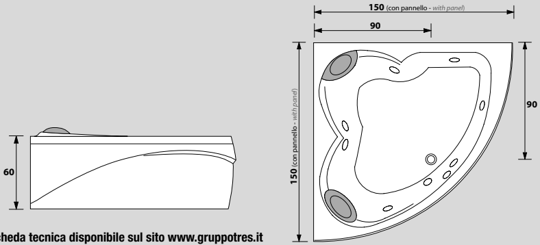
Scheda tecnica disponibile sul sito www.gruppotres.it Technical drawing available on www.gruppotres.it
