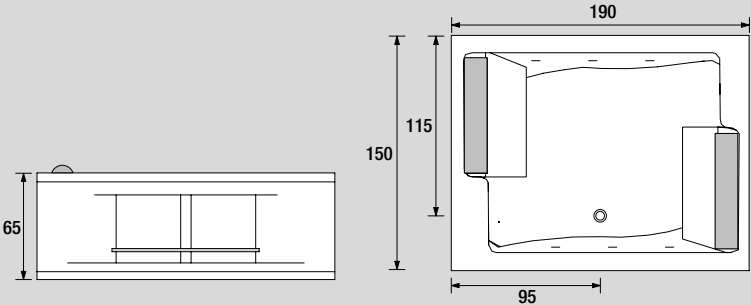
Scheda tecnica disponibile sul sito www.gruppopotres.it Technical drawing available on www.gruppopotres.it
